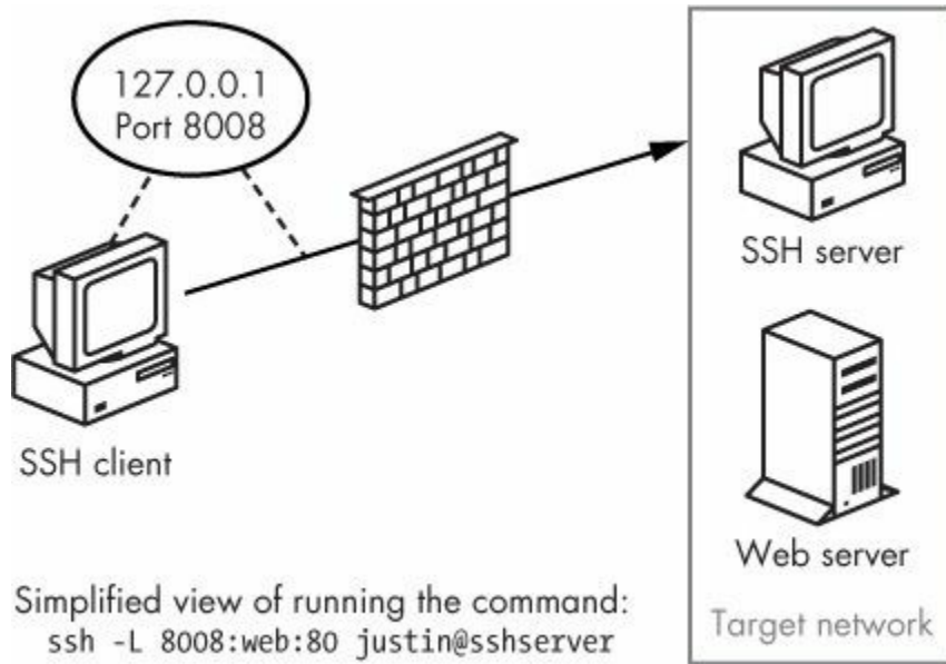
Şekil 2-2. SSH ileri tünelleme
